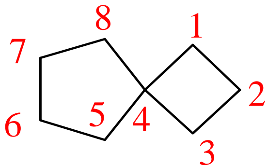
螺[3.4]辛烷 Spiro[3.4]octane
